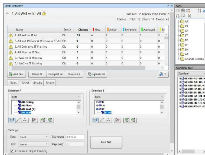
รูปที่ 2.2 หน้าต่างการทำ Clash Detection ใน Navisworks
