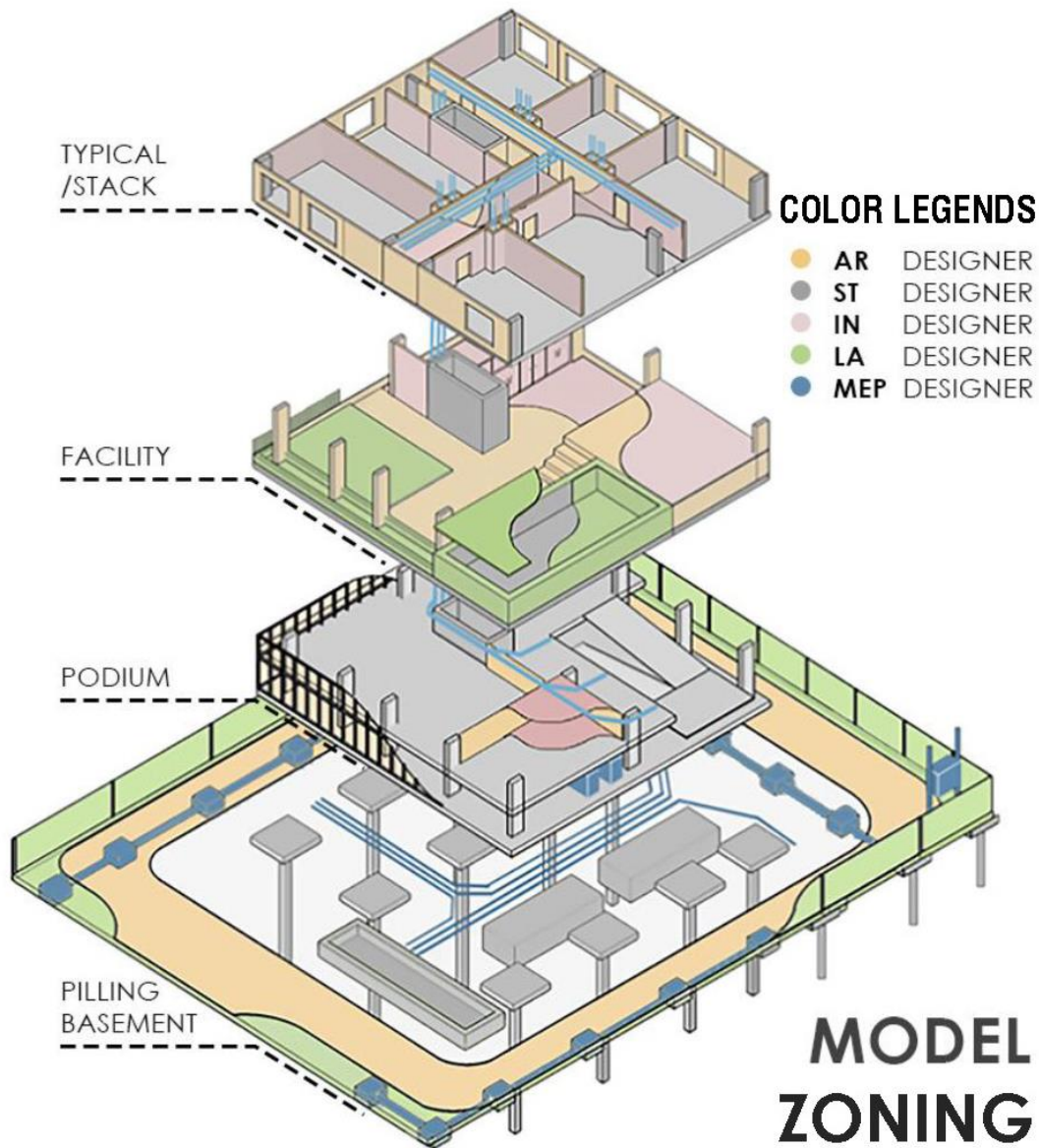
รูปที่ 3.1 Model Ownership - Zoning Diagram
